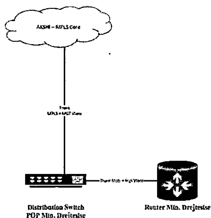
Figura nr. 4: Skema logjike e ofrimit të shërbimeve nga AKSHI
