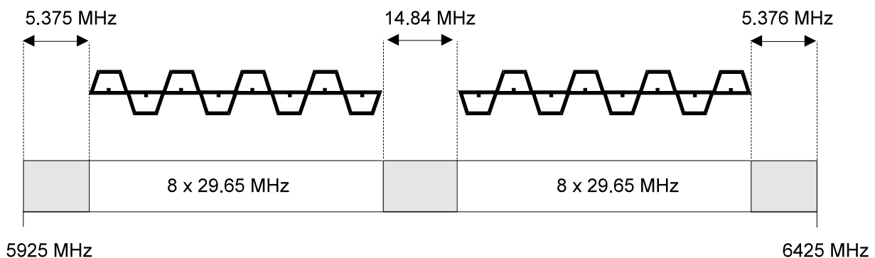
Figura 7. Ndarja e kanaleve për brezin 5925 – 6425 MHz
