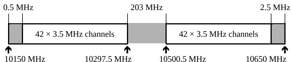
Figura 16. Brezi i frekuencave 10 – 10.68 GHz
