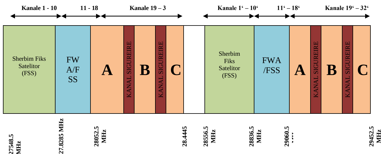
Figura 20: Plani i brezit 29 GHz
