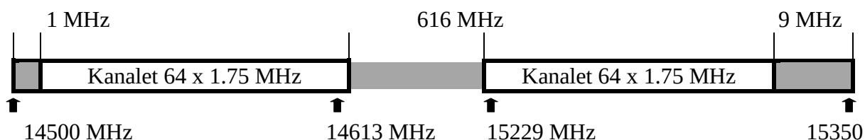
Figura 23. Brezi i frekuencave 14.5 – 15.35 GHz
