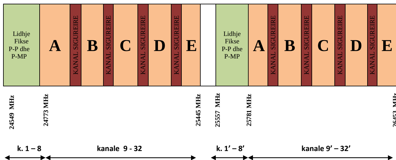
Figura : Plani i brezit 26 GHz
