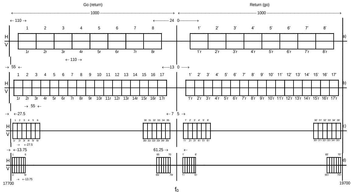
Ndarjet e kanaleve të radio- frekuencave për sistemet radio-rele që punojnë në brezin 17.7-19.7 GHz the 17.7 GHz - 19.7 GHz band (Ndarja e kanaleve)
