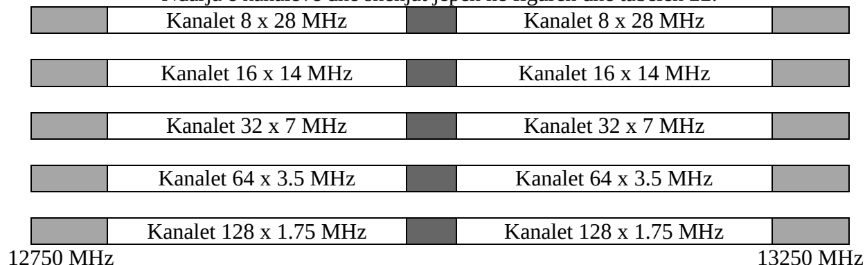
Figura 20. Brezi i frekuencave 12.75-13.25 GHz
