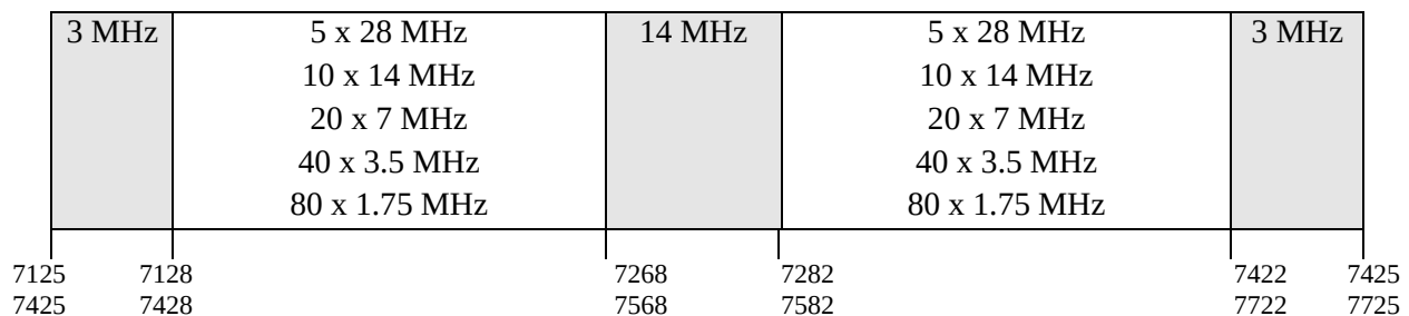
Figura 11. Brezi i frekuencave 7425 – 7725 MHz
