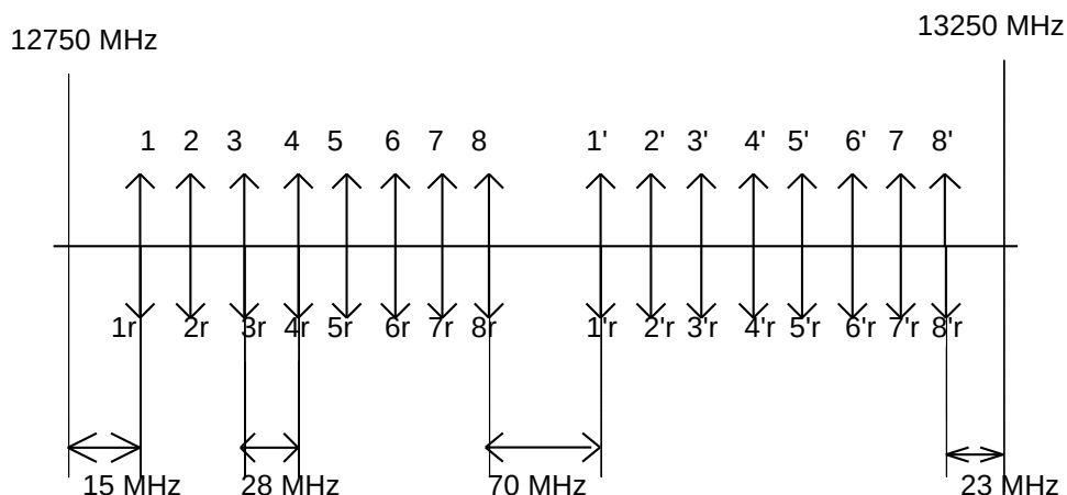
Ndarja e kanaleve të radio frekuencës duke përdorur gjerësi kanali 28 MHz
