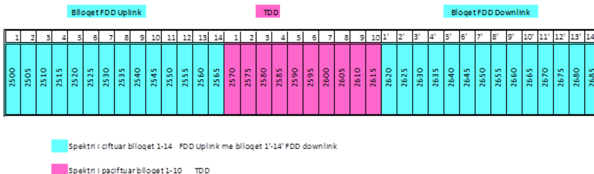
NDARJA NE BLOQE NE BREZIN 2500-2690 MHZ
