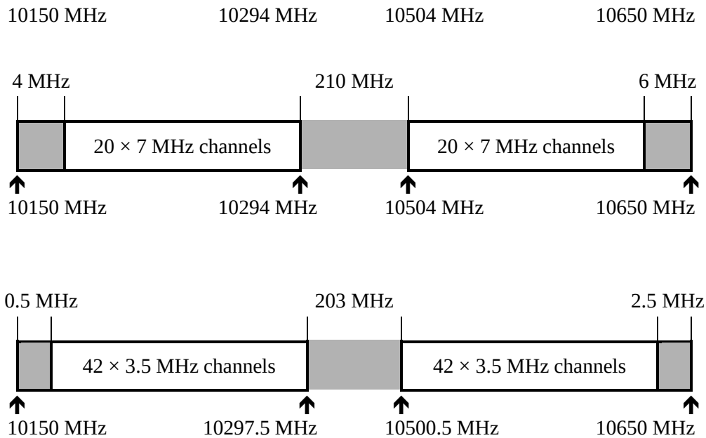
Figura 16. Brezi i frekuencave 10 – 10.68 GHz
