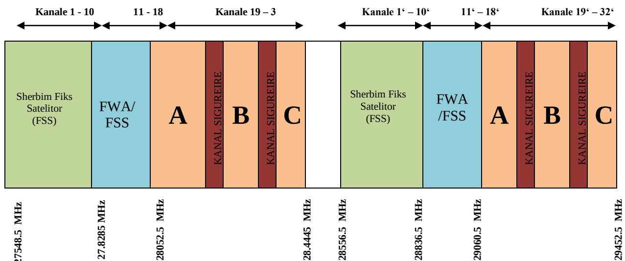
Figura 20: Plani i brezit 29 GHz
