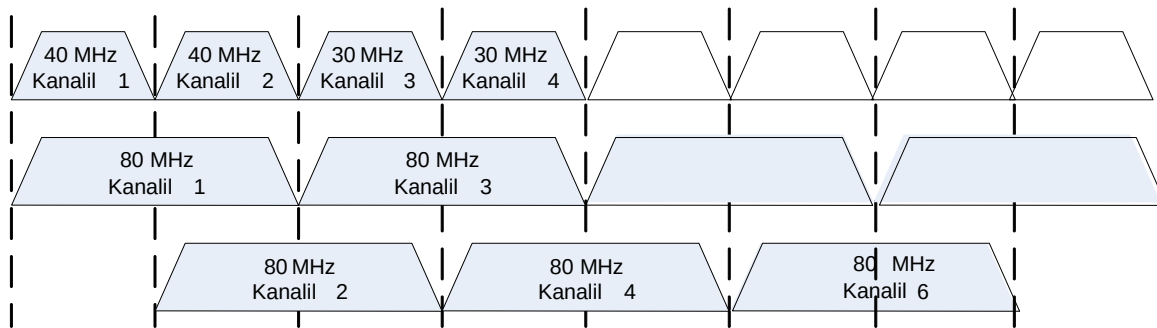
Figura 9: Ilustrimi i identifikuesve të kanalit për derivimin e kanaleve në 60MHz
