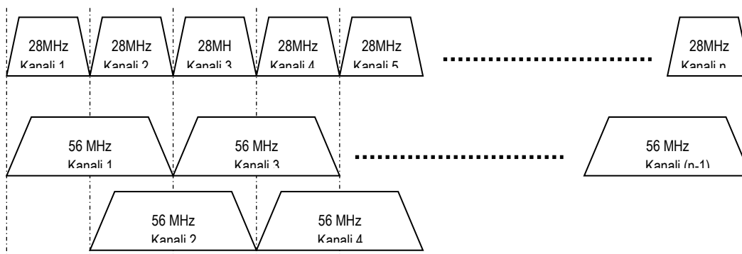
Figura 15 Identifikimi i kanaleve 56 MHz
