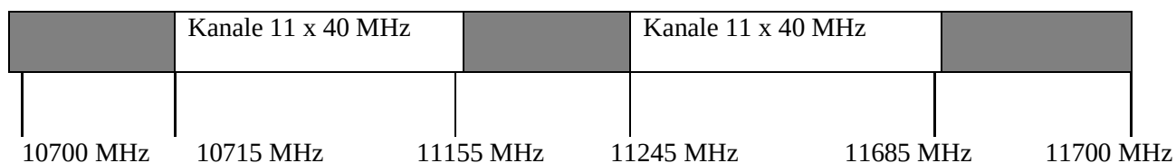
Figura 18. Ndarja e kanaleve për sistemet me gjerësi kanali 40 MHz
